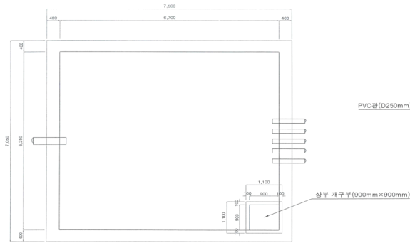
평면도
