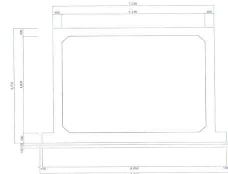
측면도 <2>
