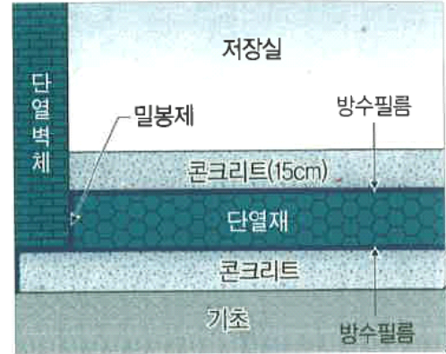
저온저장고 바닥시공 단면도
