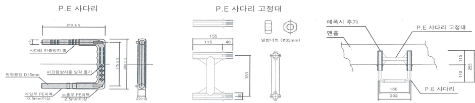
사다리 상세도
