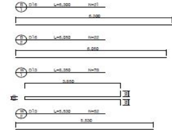
철근재료표
